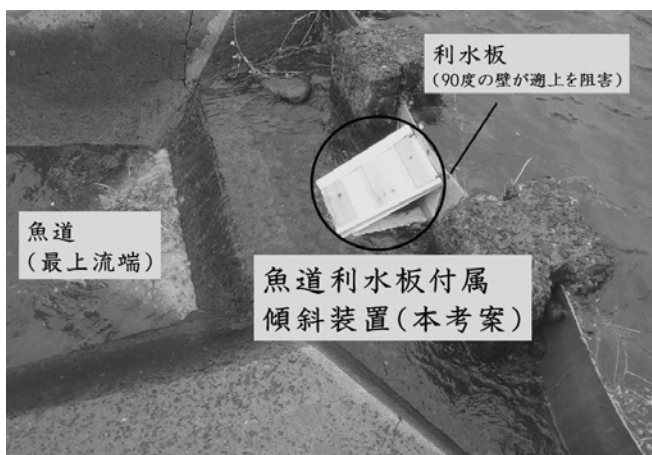
図7 魚類遡上円滑化傾斜装置
