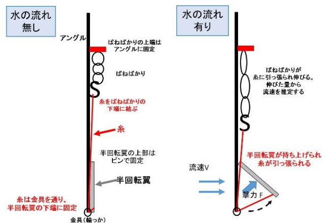
図 7 恵下の簡易型流速計の仕組み
