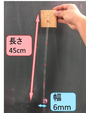
図 5 アクリル棒を使った流速計
