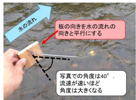
図 3 実際の測定の様子
