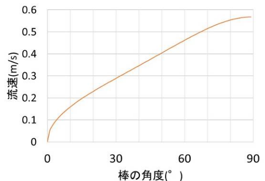
図 4 角度と流速のグラフ
